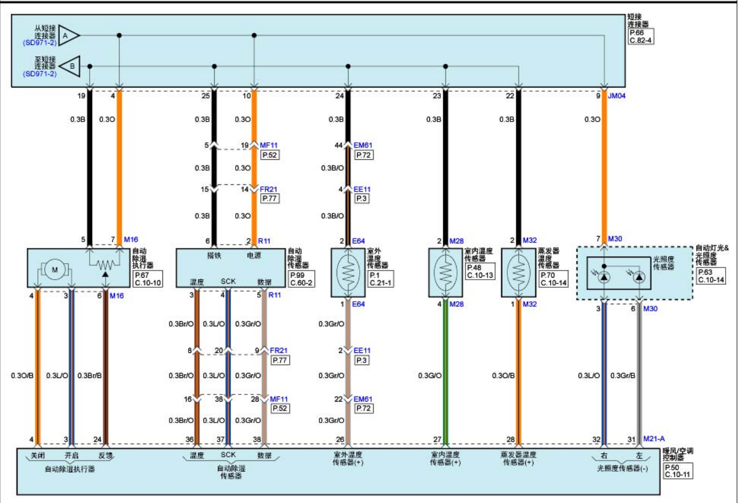
空调控制系统(自动)(3)
